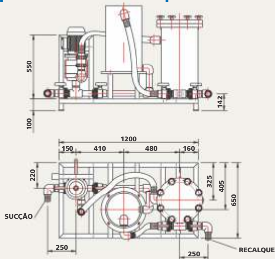
Filtro Galvânico Maxfiltro tipo disco 240 com tanque de mistura
