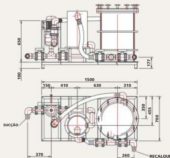
Filtro Galvânico Maxfiltro tipo disco 400 com tanque de mistura
